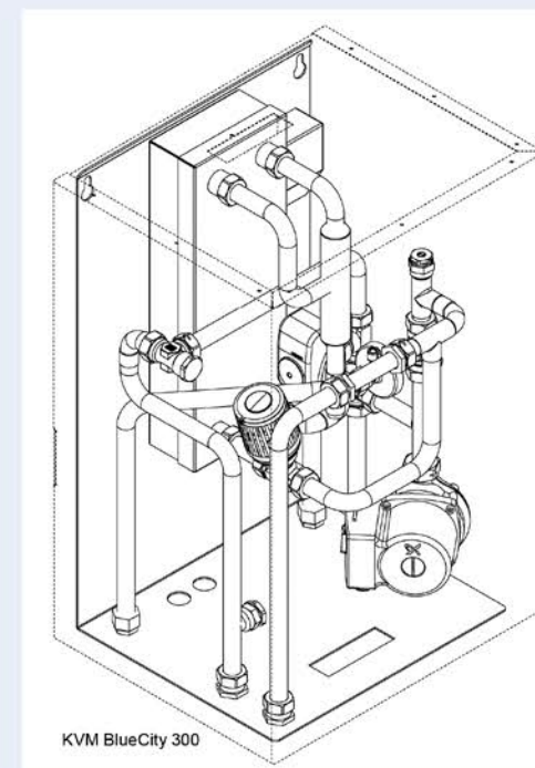
▲ Stadsverwarmingsunit Ferroli Blue City
